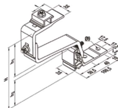
Gancio in alluminio per tegole e listelli GTLA
